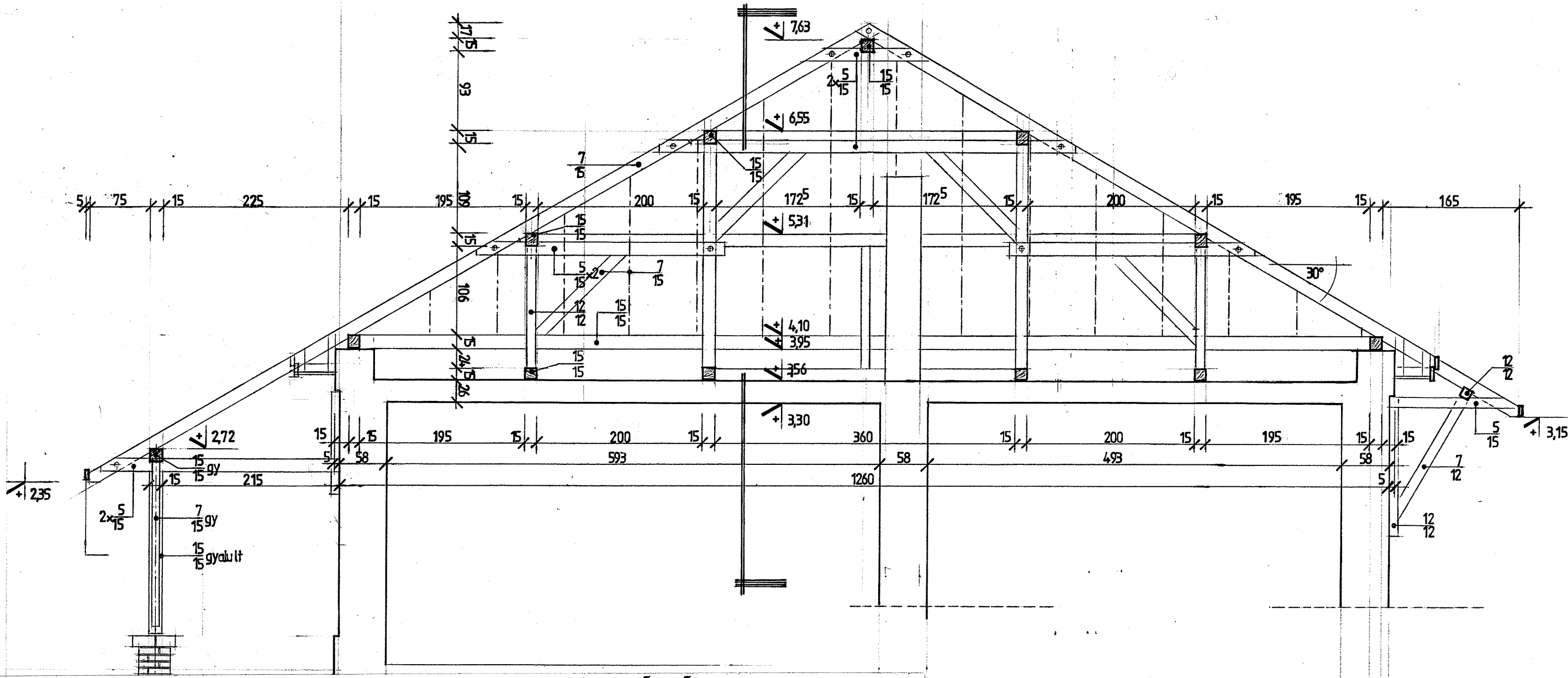
TERVEZETT B-B KERESZTMETSZETI KIALAKÍTÁS M=1:50
